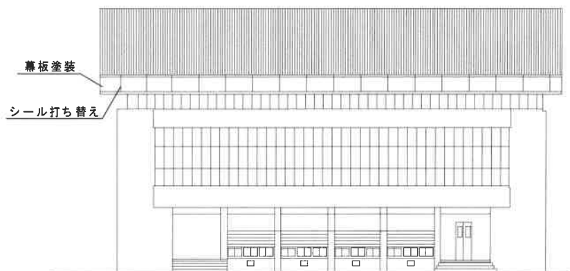
西側立面図
