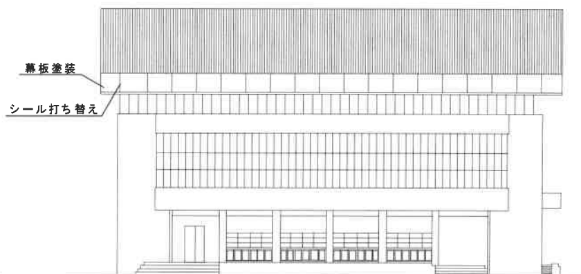
東側立面図
